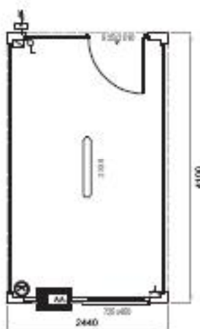
CLIP 10
